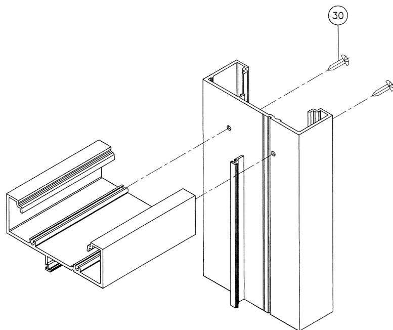
DOOR TOP CORNER
